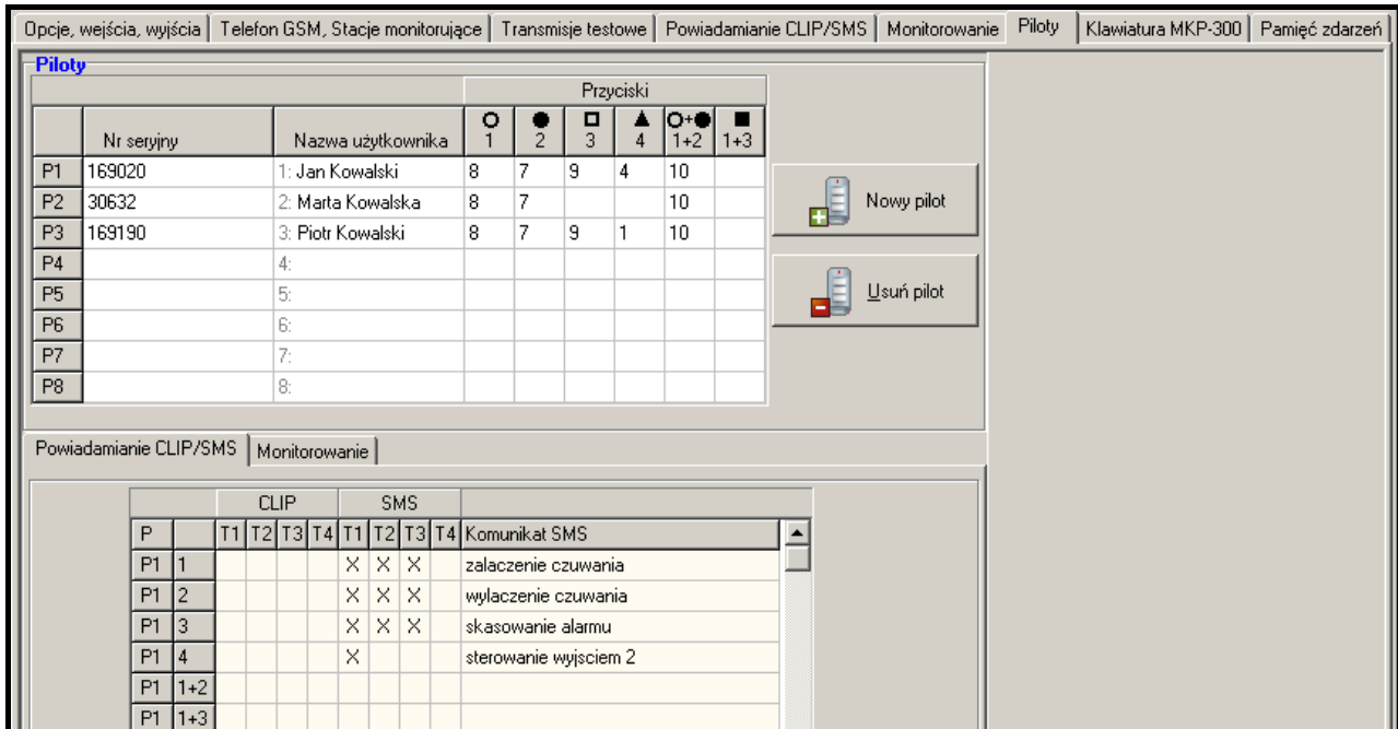
Rys. 15. Zakładka „Piloty”.
