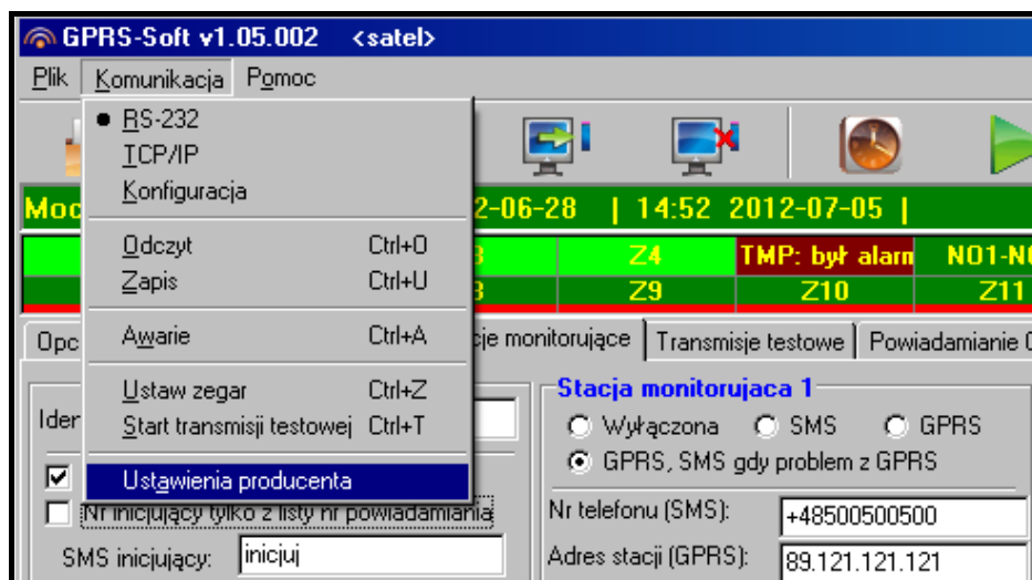
Rys. 20. Polecenie „Ustawienia producenta” w menu „Komunikacja”.
