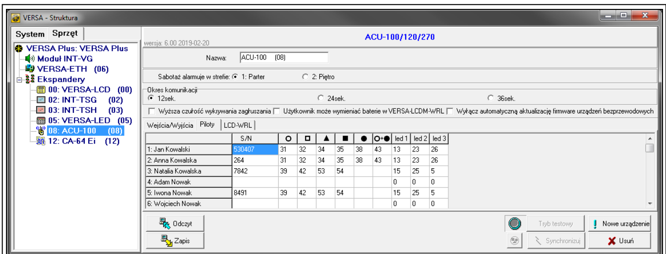
Rys. 25. Program DLOADX: zarządzanie pilotami w przypadku kontrolera podłączonego do centrali VERSA / VERSA Plus / VERSA IP.
