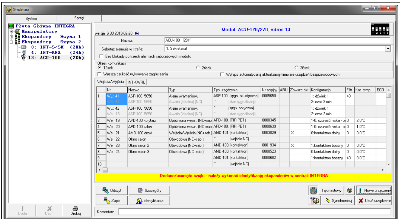
Rys. 21. Program DLOADX: informacje wyświetlane po zarejestrowaniu nowego urządzenia w kontrolerze podłączonym do centrali INTEGRA / INTEGRA Plus.
