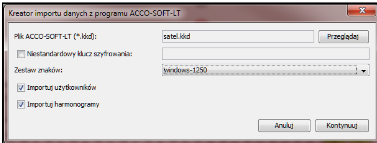
Rys. 55. Okno do importowania danych z programu ACCO-SOFT-LT.
