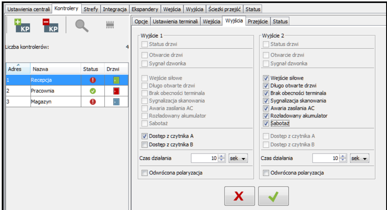
Rys. 18. Zakładka „Wyjścia”.
