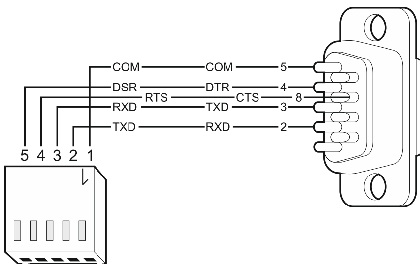
Rys. 15. Sposób połączenia portów RS-232 modułu i komputera. Po lewej wtyk PIN-5. Po prawej wtyk żeński DB-9 od strony punktów lutowniczych.
