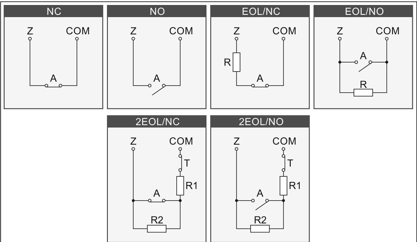
Rys. 16. Sposoby podłączania czujek do wejść. Wyjścia czujki oznaczone są literami: A - alarmowe, T – sabotażowe. R=R1+R2.
