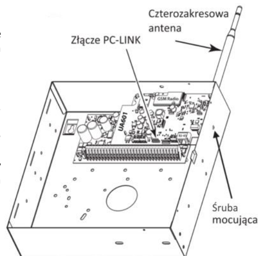
Rysunek 2 Montaż uchwytu w obudowie
