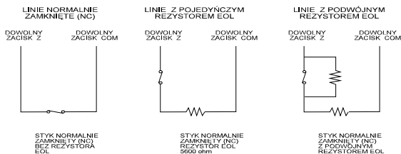
Rys. Podłączenie linii do włączania/wyłączania systemu kluczem.
