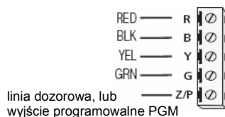
Zaciski klawiatur PK55XX/RFK55XX
