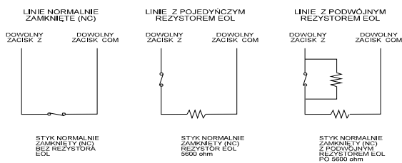
Rys. Podłączenie linii do włączania/wyłączania systemu kluczem.
