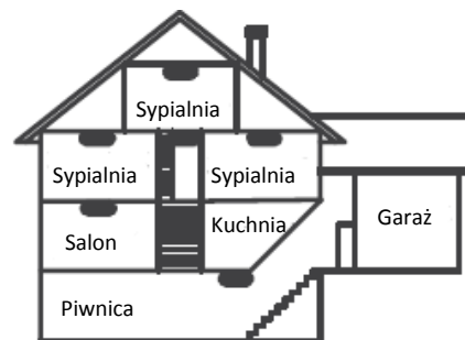
● Rozmieszczenie czujek tlenku węgla
